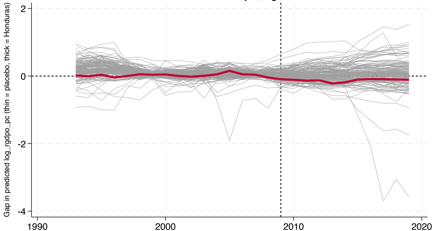
World: naive_yrs_log
